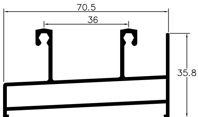
70L08 Soleira c/ caixa
