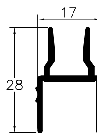
70L18 Perfil ligação 3/4 folhas
