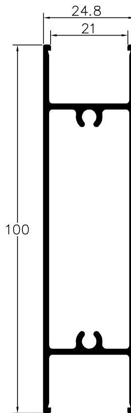
70L14 Travessa do meio
