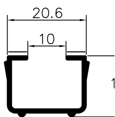
70L17 Redutor p/ vidro simples
