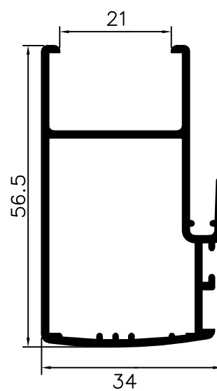
70L16 Central móvel
