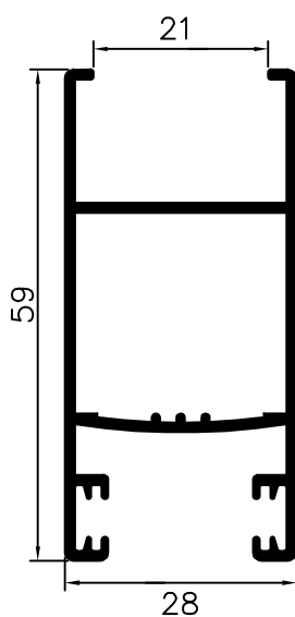
70L15 Lateral móvel
