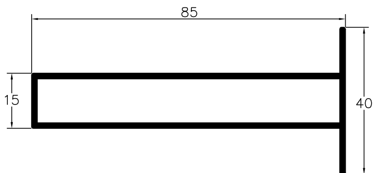
M03 Perfil ligação caixilho
