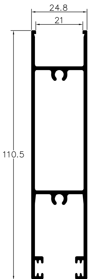
70L13 Travessa do fundo
