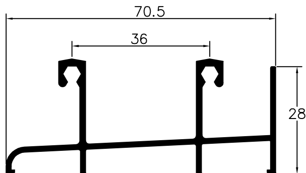
70L09 Soleira s/ caixa
