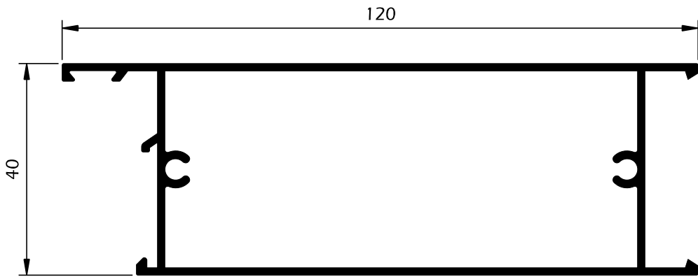
BP69 Almofada de baixo 120mm
