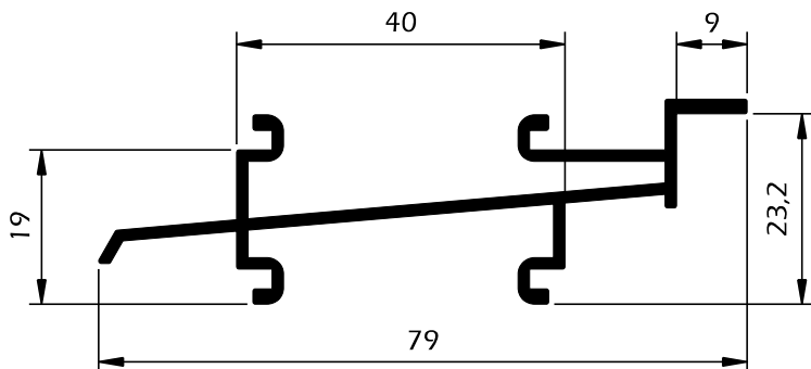
BP32 Soleira condensação
