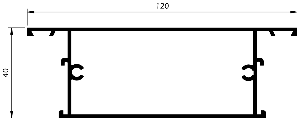
BP58 Almofada do meio 120mm
