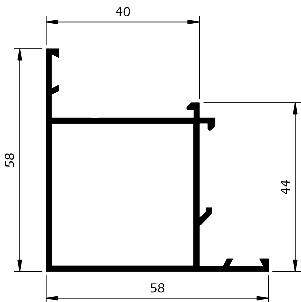
BP36 Canto reto
