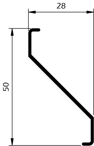
Z37 Lâmina em Z
