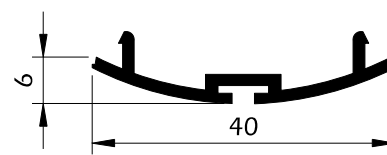
4068 Perfil p/ portas vai-vem
