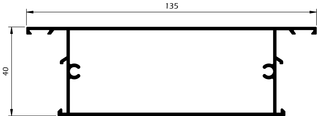
BP08 Almofada do meio 135mm
