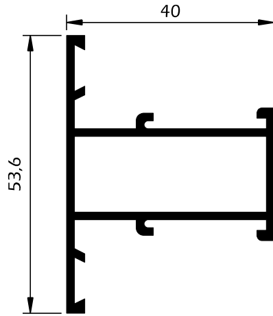
BP24 Travessa estreita s/ olhais
