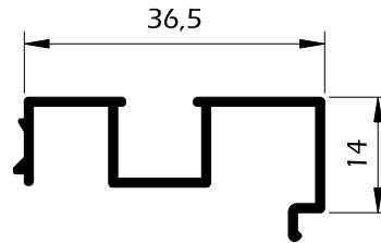
Z46 Bite para persianas
