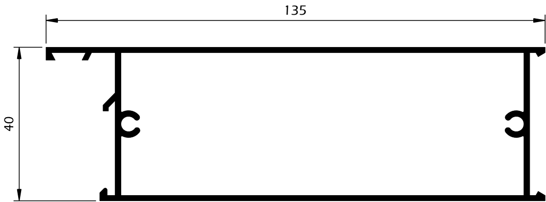
BP09 Almofada de baixo 135mm
