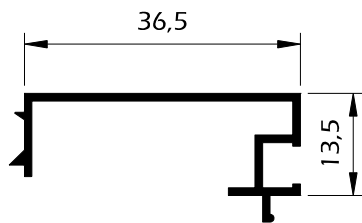
Z36 Bite para persianas
