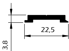
BP07 Barra de cremone
