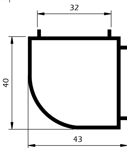
BP4098 Canto redondo 90°
