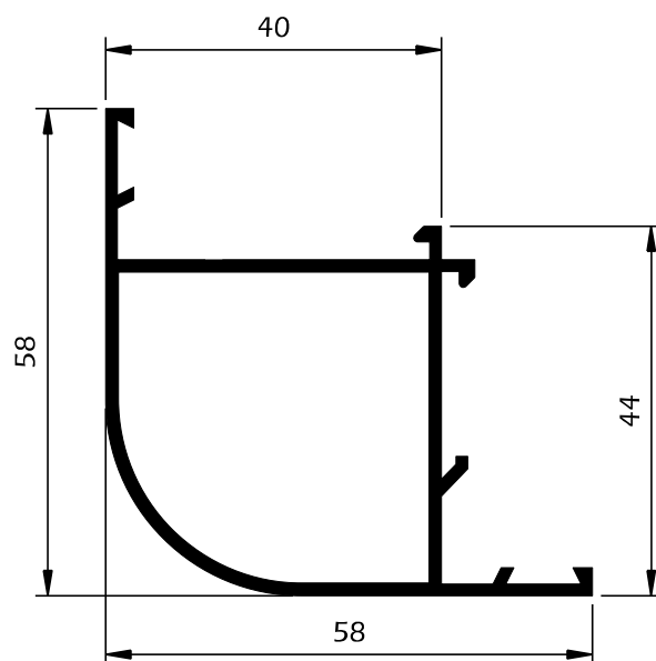
BP37 Canto redondo
