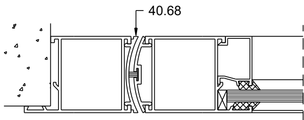
BP07 Barra de cremone
