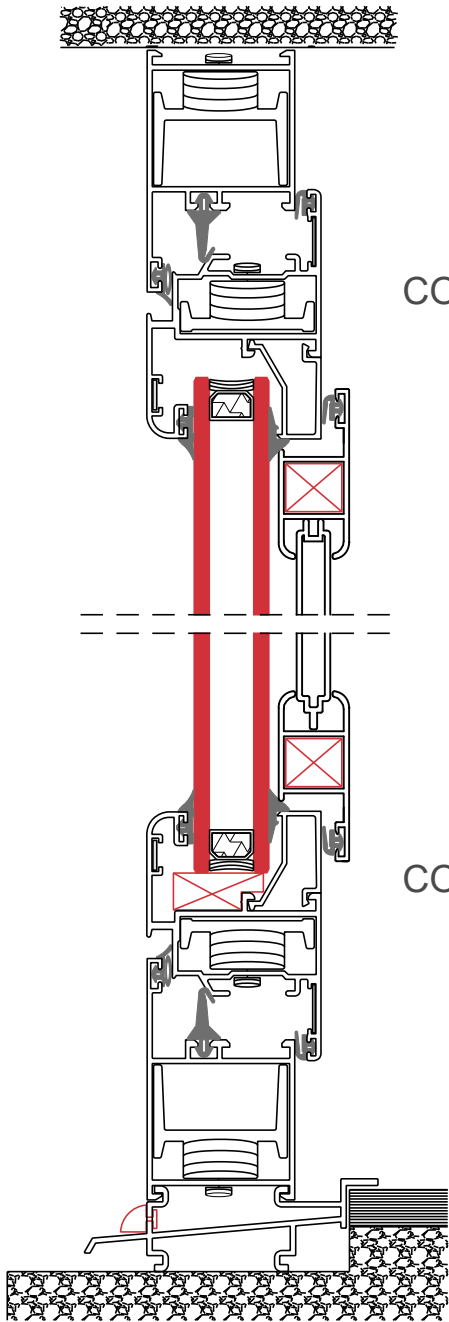
CORTE 3
