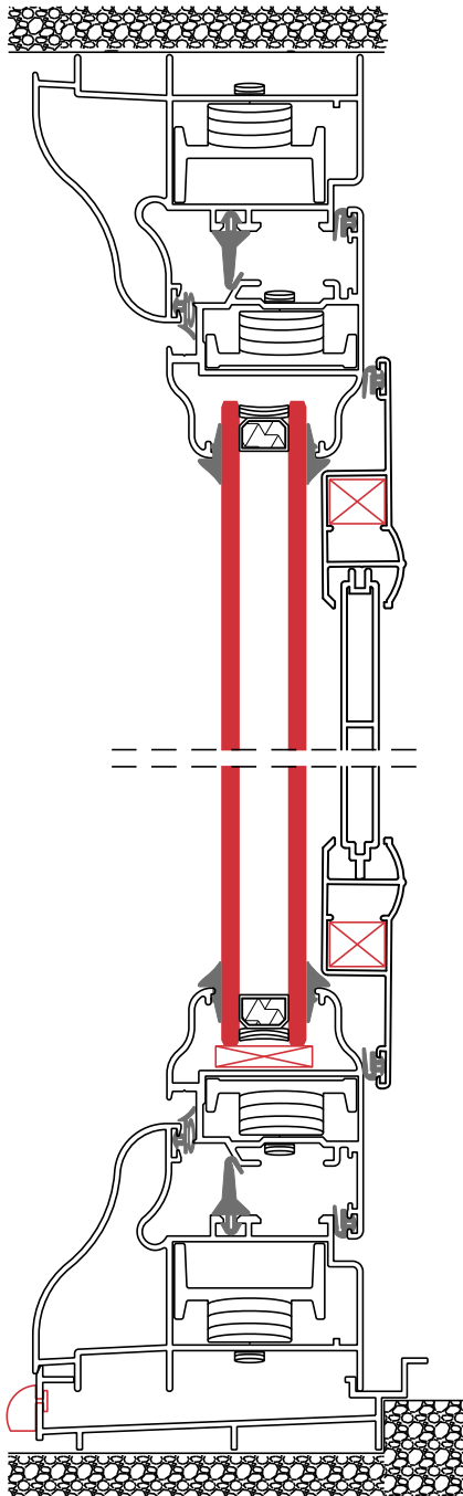
CORTE 5
